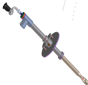
Lingl-Reingas-Injektor-Brenner (LRGIB)
