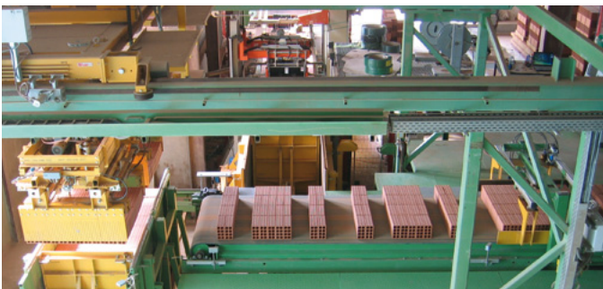
Installation de déchargement et de conditionnement Unloading and packaging installation
